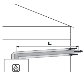
C13 Uygulama Örneği
