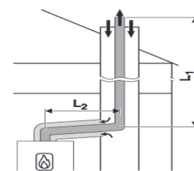
C93 Uygulama Örneği
