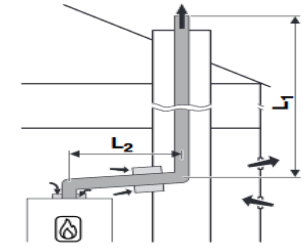
B Tipi Uygulama Örneği
