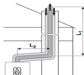
C33 Uygulama Örneği
