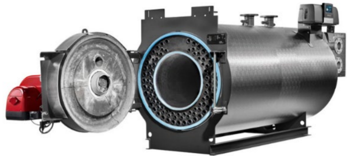
Entegre ECO Ekonomizör
