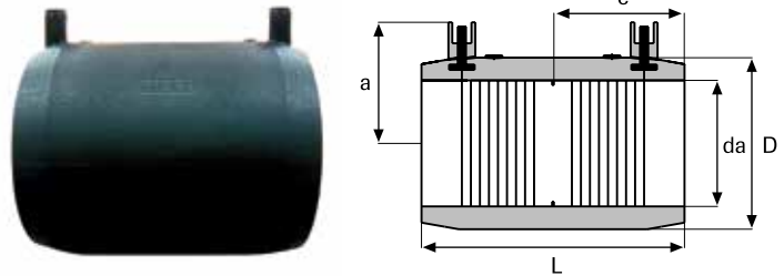
PE 100 EF Manşon Ölçü Tablosu*
